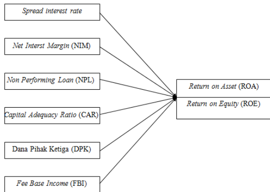
Gambar 1. Kerangka Pemikiran
